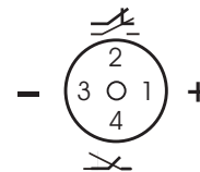
Цоколевка соединителя CS S254-3 (вид со стороны монтажа)
